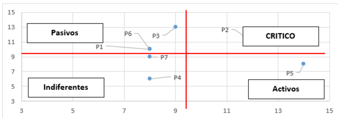
Figura 1. Gráfico de los problemas en el plano cartesiano
