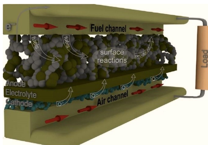
Figura 1. Celda de combustible de óxidos sólidos, Alvarado (2015).
