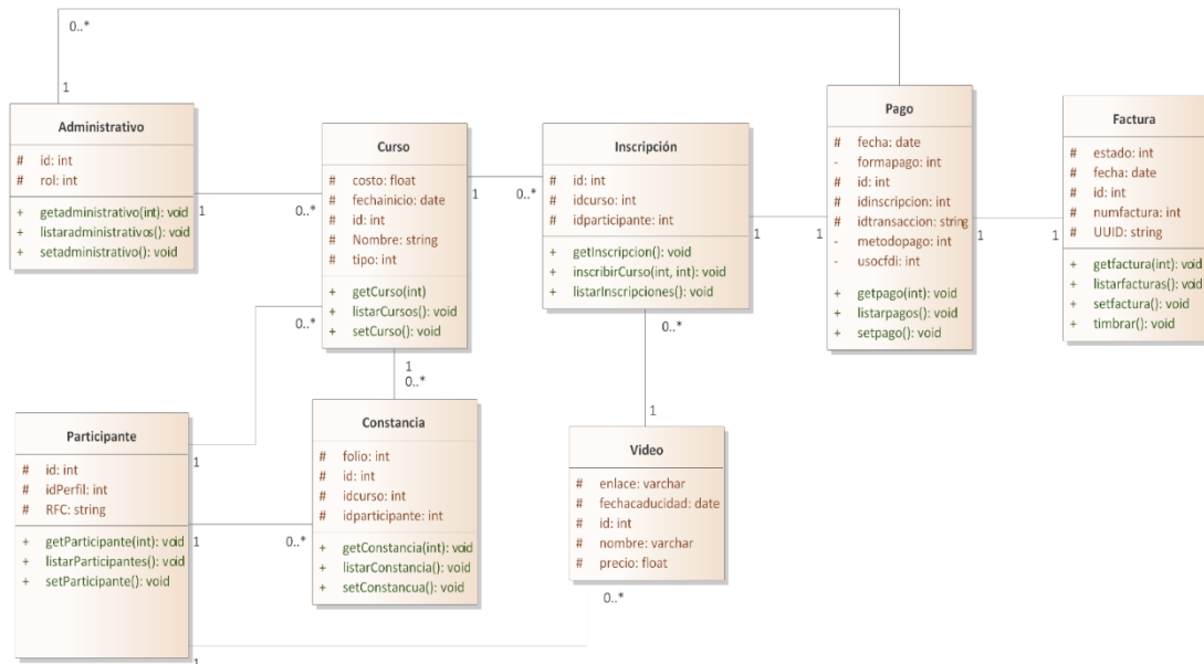
Figura 5: Diagrama de clases para el sistema de gestión de cursos para el CCPGRO
