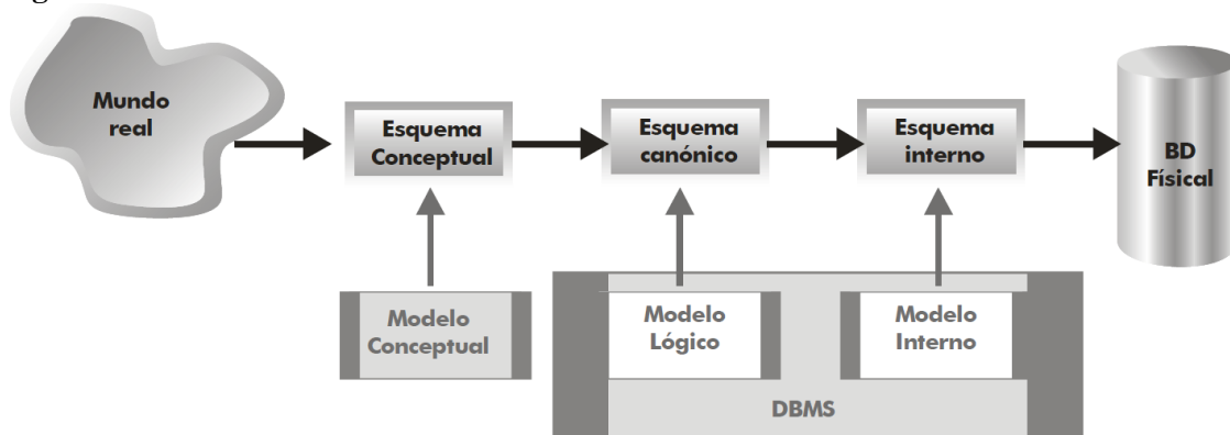
Figura 2: Clasificación de los modelos de datos
