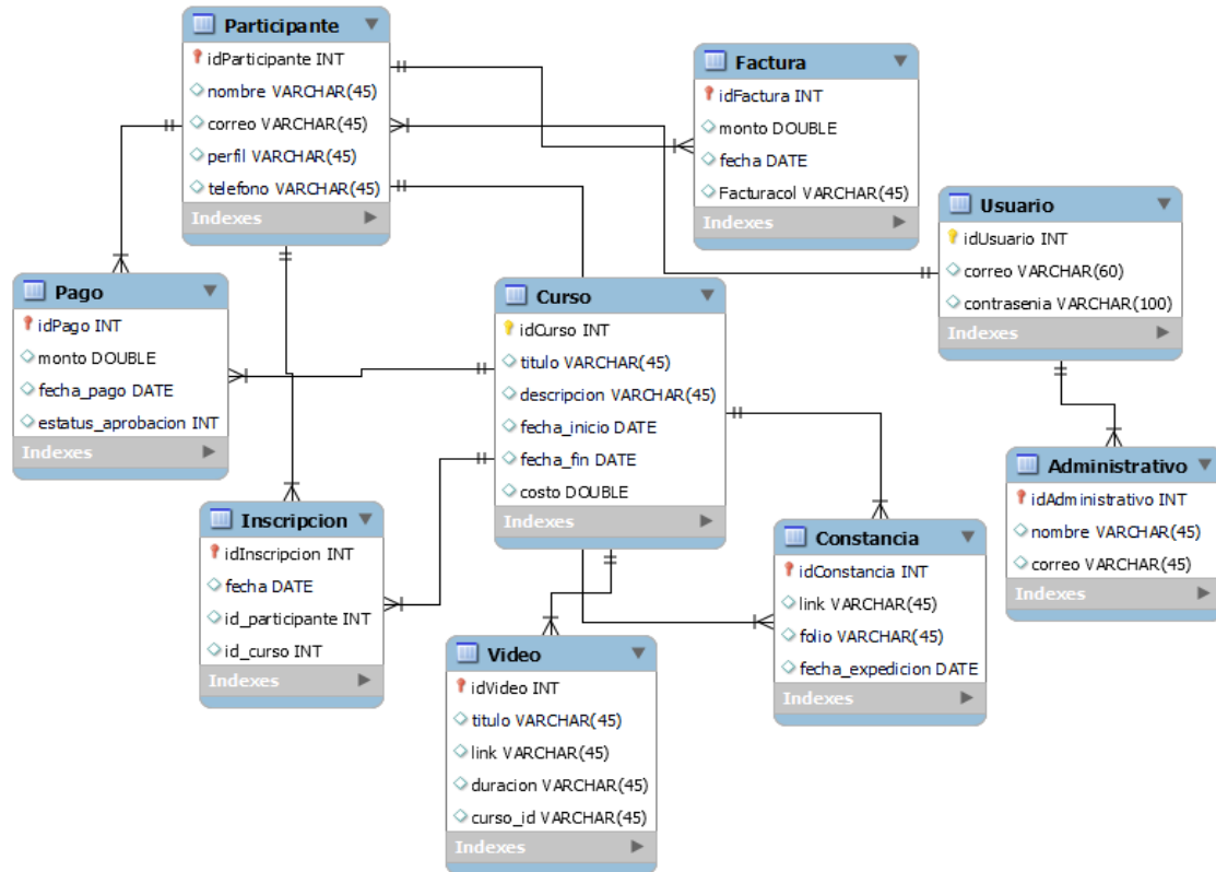
Figura 6: Diagrama entidad-relación para el sistema de gestión de los cursos en línea que ofrece el CCPGRO.
