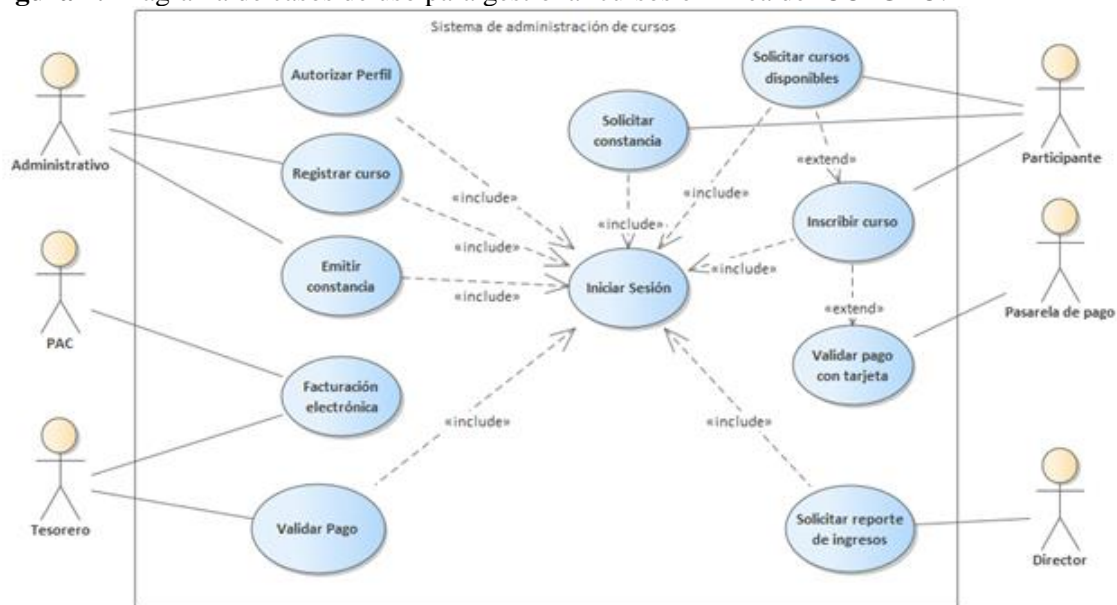
Figura 4: Diagrama de casos de uso para gestionar cursos en línea del CCPGRO.
