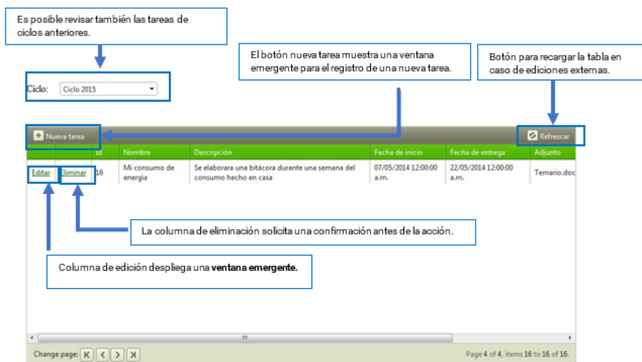
Figura 14. Descripción de campos para la tabla de “Tareas”.
