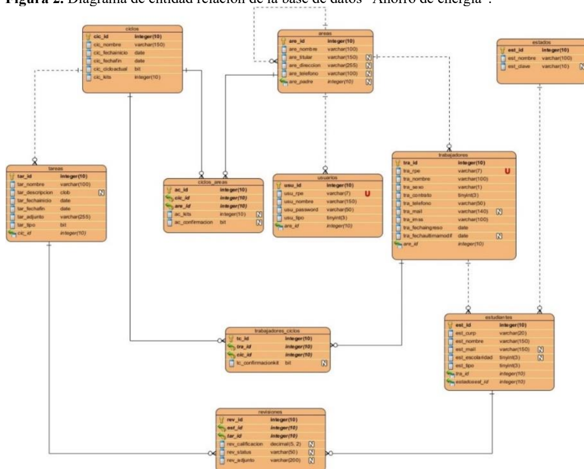
Figura 2. Diagrama de entidad relación de la base de datos “Ahorro de energía”.
